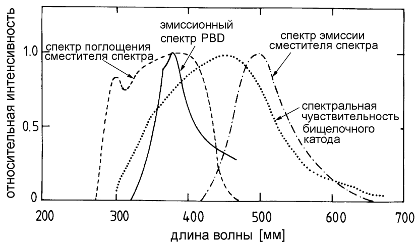
Рис. 5.10: Эмиссионные спектры первично флуоресцирующего материала (PBD) и сместителя спектра (BQ) в сравнении с спектральными чувствительностями фотокатодов для обычно используемых фотоумножителей [1,395].
