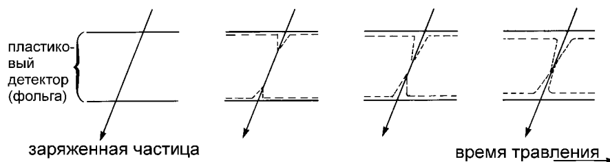
Рис. 4.96: Развитие во времени конусов травления в пластиковом детекторе.
