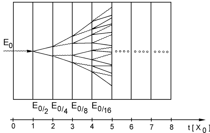
Рис. 7.24: Простая модель параметризации ливня
