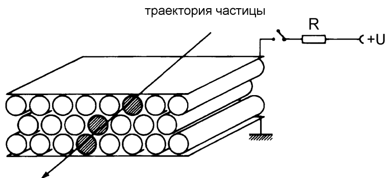
Рис. 4.77: Принцип действия камеры на разрядных трубках.
