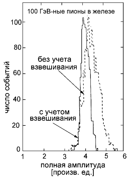
Рис. 7.45: Амплитудное распределение для пионов с энергией 100 ГэВ в железном калориметре на стримерных трубках с и без весовых факторов [518]. Весовой фактор был оптимизирован для начальной энергии 100 ГэВ.
