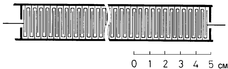
Рис. 4.19: Структура катода в виде меандра, используемая в качестве линии задержки для считывания координаты вдоль анодной проволоки в стримерной трубке [165].
