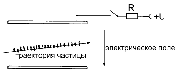
Рис. 4.72: Принципиальное устройство стримерной камеры.
