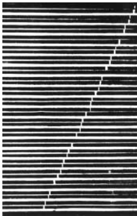
Рис. 4.82: Трек космического мюона в многопластинчатой искровой камере [339].
