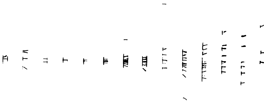
Рис. 4.84: Фотография электронного каскада в многопластинчатой стеклянной искровой камере [343–345].
