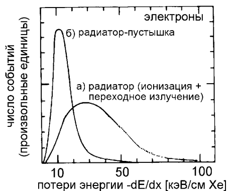
Рис. 6.23: Типичное распределение потерь энергии для электронов высокой энергии в детекторе переходного излучения с а) реальным радиатором и б) радиатором-пустышкой [450].
