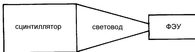
Рис. 5.13: Собираение света с помощью световода типа «рыбий хвост».
