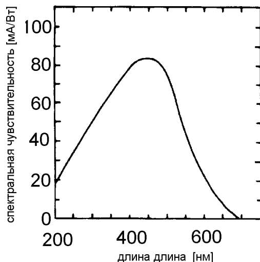
Рис. 5.4: Спектральная чувствительность бищелочного фотокатода в фотоумножителе с окном из силиката бора [379].
