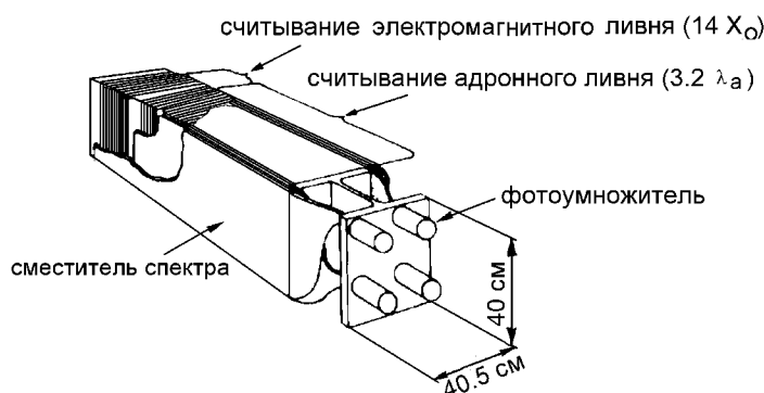
Рис. 7.30: Типичная схема калориметра на железе и скintилляторе со считыванием с помощью спектросместителей [540].
