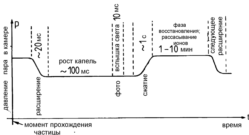
Рис. 4.69: Циклы расширения в камере Вильсона [2].
