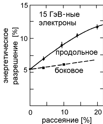
Рис. 7.25: Влияние продольных и поперечных утечек на энергетическое разрешение [9, 521].
