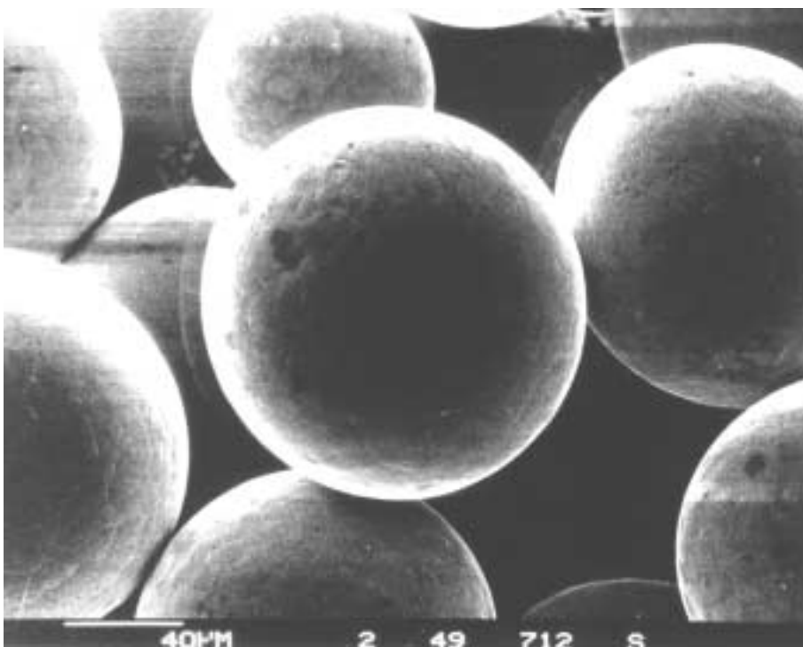
Рис. 7.56: Оловянные гранулы (диаметр = 130 мкм) в качестве криогенного калориметра. Поглощение при низкой энергии может нагреть гранулы на величину, достаточную чтобы вызвать переход из сверхпроводящего состояния в состояние с нормальной проводимостью, обеспечивая тем самым регистрируемый сигнал [590,597].
