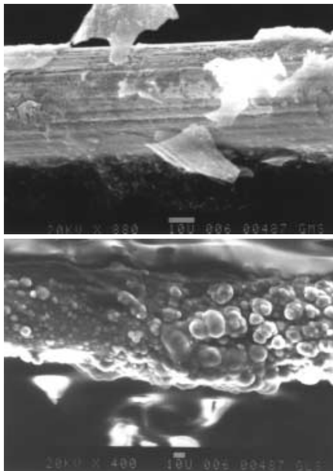
Рис. 4.63: Отложения на проволочках при старении камеры [294]: а) кремниевые на анодной проволочке ( \phi = 30 мкм); б) из кремния, хлора и меди на катодной проволочке ( \phi = 100 мкм) [294]
