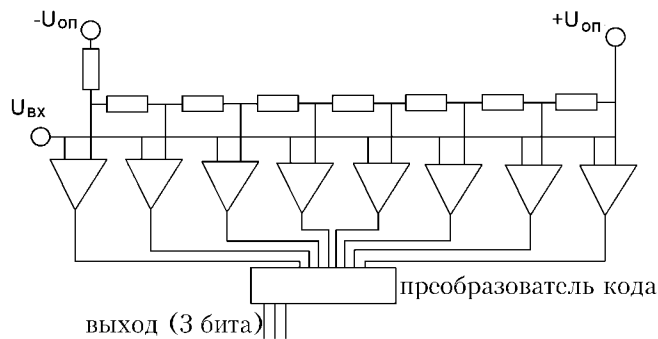
Рис. 9.7: 3х-битовый ИАЦП [603].
