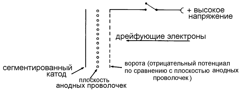
Рис. 4.58: Принцип работы «ворот» для времяпроекционной камеры.
