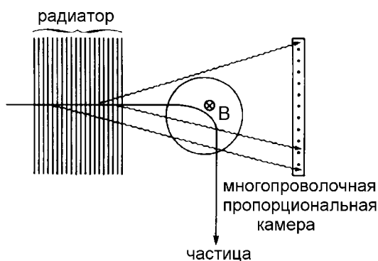
Рис. 6.24: Изучение эффекта образования переходного излучения без помех от налетающей частицы путем отклонения ее в магнитном поле.
