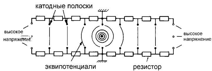
Рис. 4.36: Формирование поля в большой дрейфовой камере.
