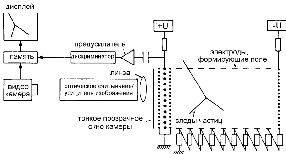
Рис. 4.61: Принцип работы камеры с оптическим съемом
