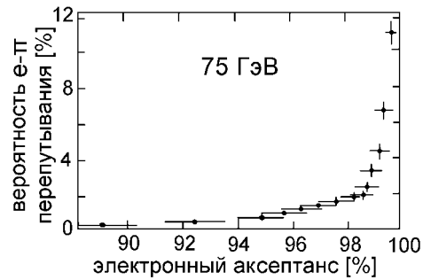
Рис. 7.50: Вероятность неправильного разделения электронов и пионов в калориметре на стримерных трубках [519,549]. Электронный акцептанс — это доля электронов, которая остается после обрезания в распределении вероятностей. Соответственно, неправильная идентификация пионов дается долей воспринятых кандидатов в электроны, которые на самом деле являются пионами.
