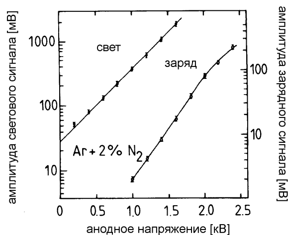
Рис. 5.11: Световой и зарядовый сигналы в газовой сцинтилляционной дрейфовой камере, заполненной аргонем с 2%-ной добавкой азота ( N_2 ), при облучении ее \alpha -частицами из ^{241}Am -источника [401]. Абсолютные амплитуды светового и зарядового сигналов несопоставимы, так как получены с использованием различных электронных систем считывания.
