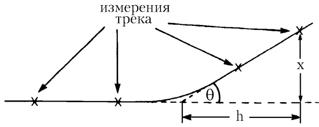
Рис. 8.3: Схема, иллюстрирующая определение ошибок трековых измерений.
