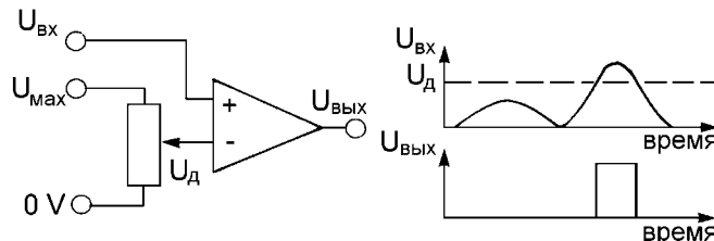
Рис. 9.3: Пороговый дискриминатор с уровнем U_d перенастраиваемым от 0В до U_{max} [603].
