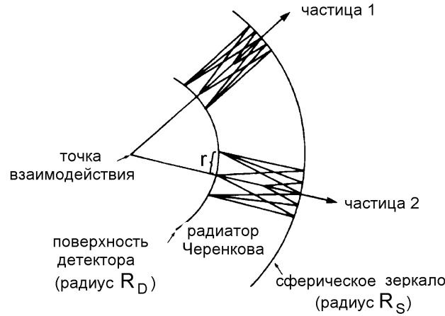
Рис. 6.14: Принцип работы черенковского счетчика кольцевого изображения (RICH) [450].
