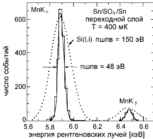
Рис. 7.13: Амплитудное распределение рентгеновских K_{\alpha} - и K_{\beta} -линий (марганец) в переходном слое Sn/SO x /Sn. Для сравнения пунктирной линией показано самое лучшее разрешение, достигнутое на Si(Li) полупроводниковом счетчике [491].
