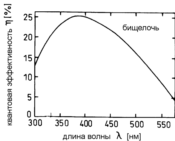
Рис. 5.2: Зависимость квантовой эффективности бищелочных катодов от длины волны света [378].
