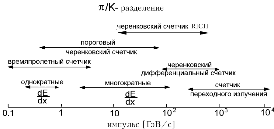
Рис. 6.34: Иллюстрация различных методов идентификации для разделения пионов и каонов вместе с характерными диапазонами импульсов.
