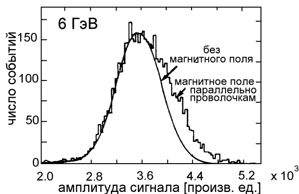
Рис. 7.54: Зависимость амплитуды сигнала от магнитного поля для электронов с энергией 6 ГэВ в калориметре на стримерных трубках [522].
