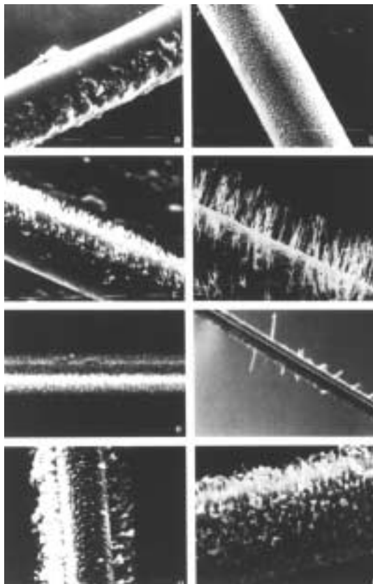
Рис. 4.62: Примеры отложений на анодных проволочках.
