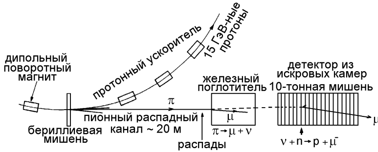
Рис. 11.10: Рождение пучка нейтрино на 15 ГэВ-ном протонном синхротроне AGS [653].
