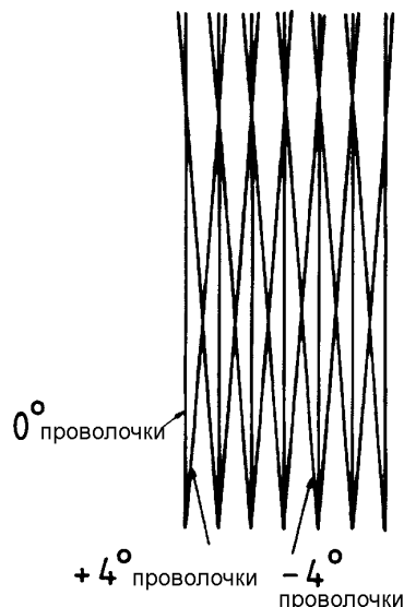
Рис. 4.45: Определение координаты вдоль анодной проволочки с использованием стерепроволочек.
