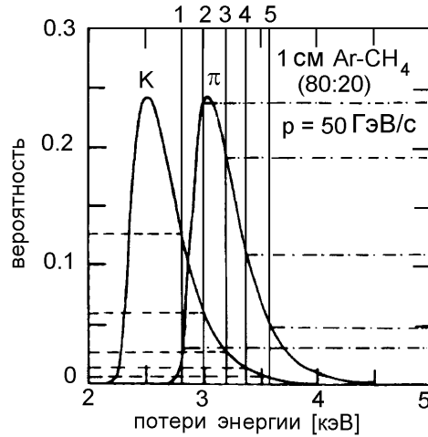
Рис. 6.32: \pi/K -разделение, основанное на распределении Ландау, проиллюстрированное пятикратным измерением потерь энергии. Указаны пять измерений dE/dx с соответствующими вероятностями P_\pi^i и P_K^i .
