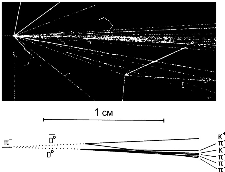
Рис. 4.67: Рождение и распад очарованных мезонов (рождение D^0 \bar{D}^0 ) в пузырьковой камере с высоким разрешением [304].
