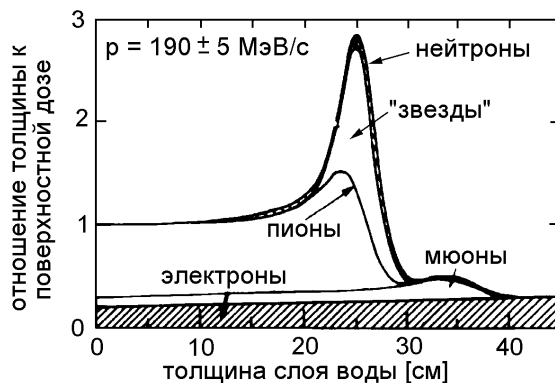
Рис. 11.5: Распределение поглощения энергии по глубине для \pi^- мезонов, мюонов и электронов [637,645].
