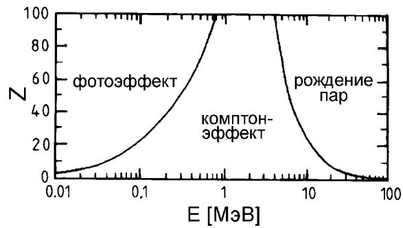
Рис. 1.15: Диапазоны энергии, в которых доминируют фотоэлектрический эффект, комптон-эффект, а также рождение пар, как функция энергии фотона и Z вещества [37,65,68].
