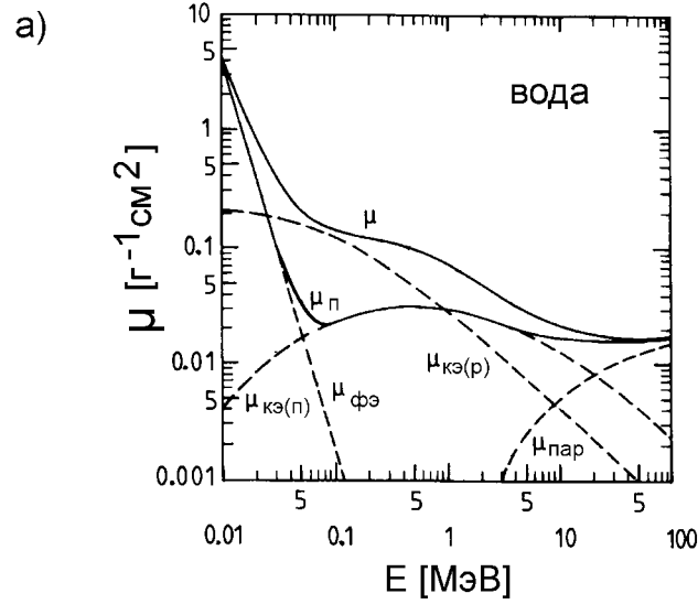
Рис. 1.14а: энергетическая зависимость массового коэффициента ослабления \mu и массового коэффициента поглощения \mu_p для фотонов в воде [63,73–75].
