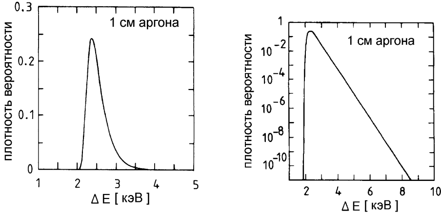
Рис. 1.3: Распределение Ландау для потерь энергии на ионизацию для 250 МэВ-ных электронов в газообразном аргоне толщиной 1 см в линейном и полупологарифмическом масштабах.
