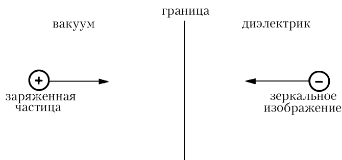
Рис. 6.20: Иллюстрация образования переходного излучения на границе сред.
