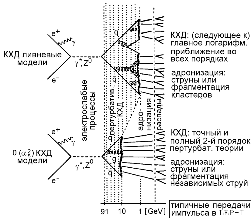
Рис. 10.5: Иллюстрация пертурбативной КХД и адронизации для реакции e^+e^- \rightarrow Z^0 \rightarrow \dots . Указаны различные фазы процесса: электрослабые взаимодействия, пертурбативная КХД, адронизация и распад частиц [620].
