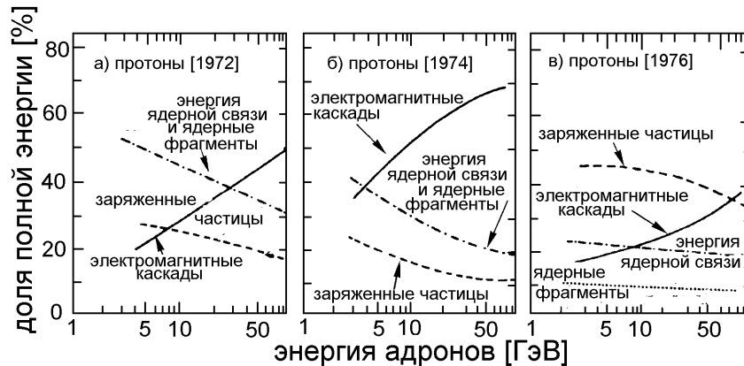
Рис. 7.35: Относительные доли энергии в адронном каскаде как функция энергии адрона [58,543–546].
