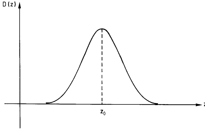
Рис. 2.2: Нормальное распределение (гауссовское распределение вокруг среднего значения z_0 ).
