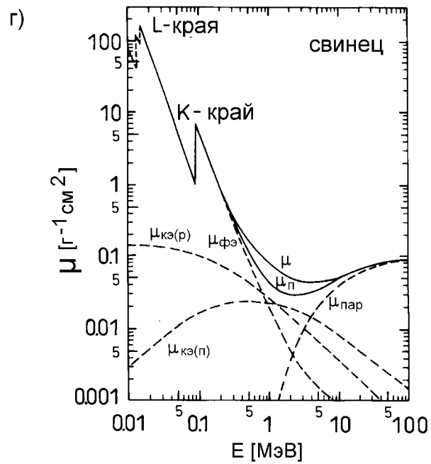
Рис. 1.14г: энергетическая зависимость массового коэффициента ослабления \mu и массового коэффициента поглощения \mu_{\text{п}} для фотонов в свинце [63,73–75].
