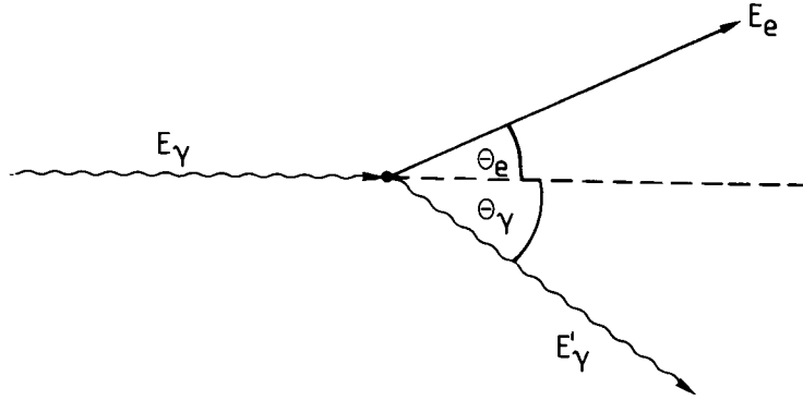
Рис. 1.12: Определение кинематических переменных при комптоновском рассеянии.
