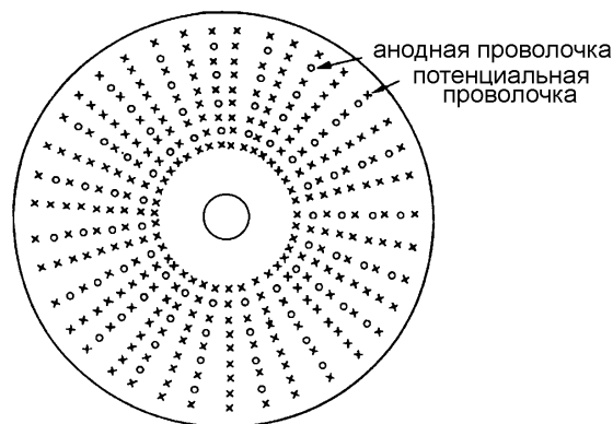
Рис. 4.41: Схематическое изображение цилиндрической дрейфовой камеры. На рисунке показан вид камеры перпендикулярно проволочкам.
