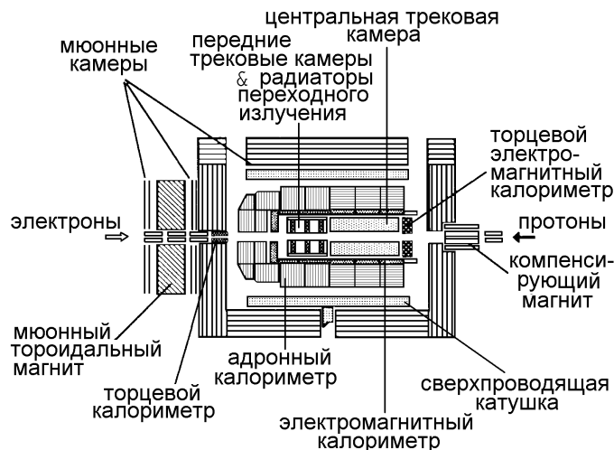
Рис. 9.8: Детектор H1 [605,606].
