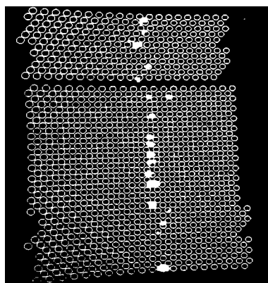
Рис. 5.17: Трек заряженной частицы в стопке сцинтилляционных волокон. Диаметр волокна до 1 мм [416].
