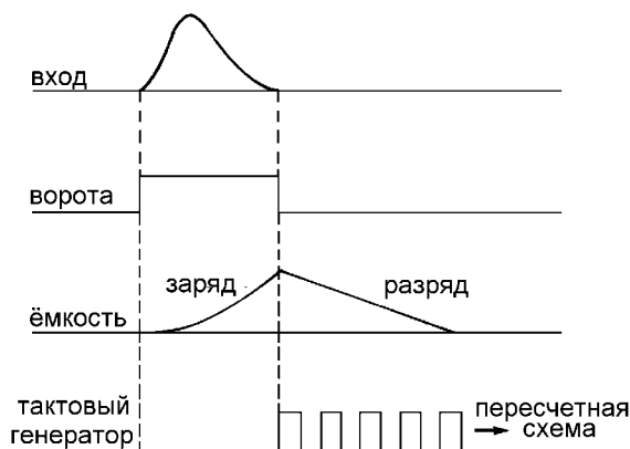
Рис. 9.5: Принцип работы ЗЦП [7].
