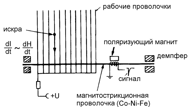
Рис. 4.86: Принцип магнестрикционного считывания в проволочной искровой камере [104,346].
