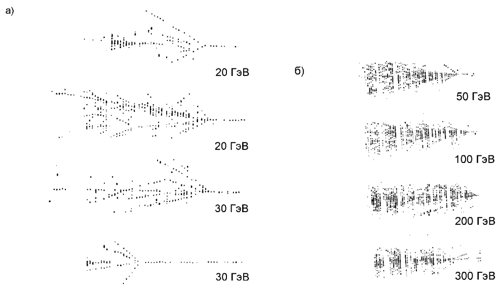
Рис. 7.42: Картина отдельных адронных каскадов с энергией 20 и 30 ГэВ (а), и 50 ÷ 300 ГэВ (б) в калориметре на разрядных камерах [560,561].
