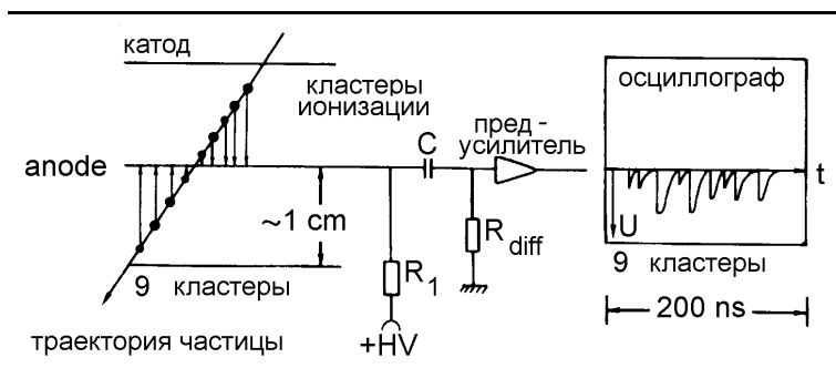
Рис. 4.11: Схема временной структуры сигнала в пропорциональном счетчике.
