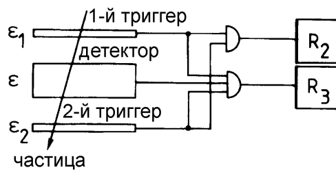
Рис. 2.5: Схема эксперимента по определению эффективности детектора.
