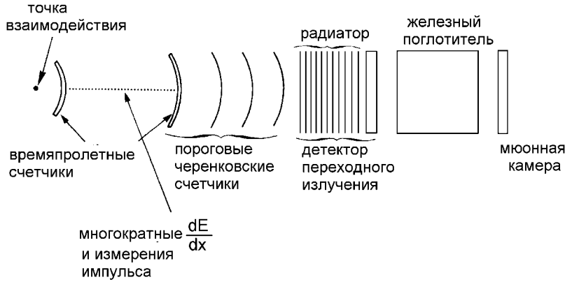
Рис. 6.35: Схема специализированного детектора для идентификации частиц.
