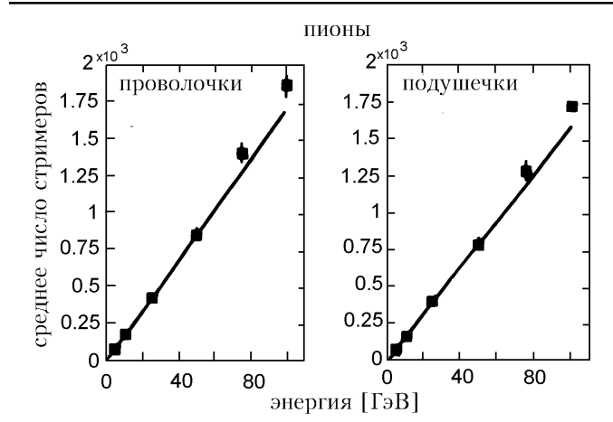
Рис. 7.44: Линейное соотношение между числом родившихся частиц и начальной энергией в железном калориметре на стримерных трубках. Показаны результаты для считывания с проволочек и подушечек [523].
