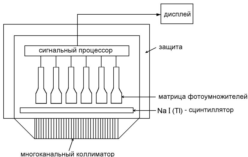
Рис. 11.1: Схематическое изображение «γ-камеры» большой площади.
