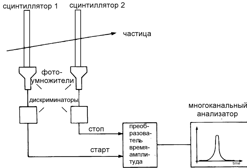
Рис. 6.5: Принцип работы времяпролетного счетчика.
