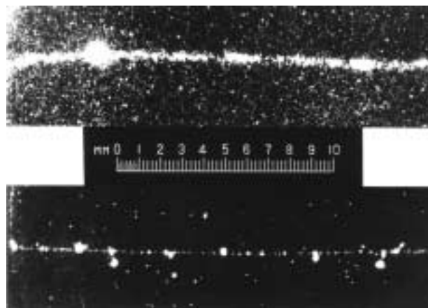
Рис. 4.76: Пример подавления диффузии в электронном треке в стримерной камере. В верхнем треке диффузия не подавлена. Она была зарегистрирована в неон-гелиевой смеси под давлением 33 атмосферы. В нижнем треке диффузия была подавлена с помощью добавления кислорода ( \approx 275 мбар) [323].
