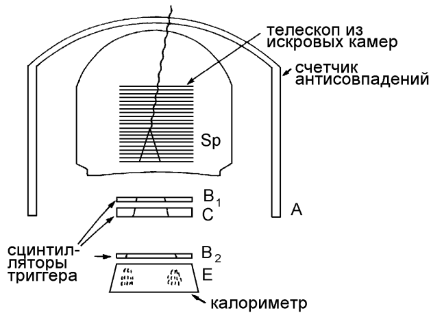
Рис. 11.13: Схема фотонного детектора для \gamma -астрономии в 100 МэВ-ном диапазоне [658, 659].
