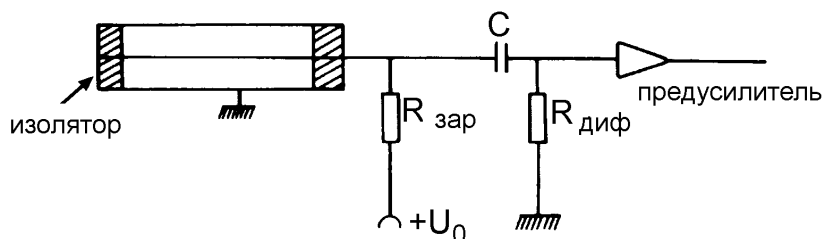
Рис. 4.10: Считывание с пропорционального счетчика.
