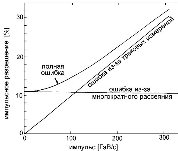
Рис. 8.6: Импульсное разрешение железного магнитного спектрометра.
