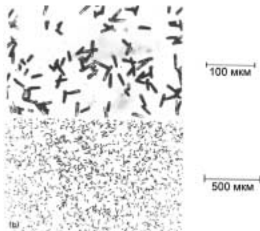
Рис. 4.98: Треки фрагментов деления в пластиковом детекторе [372]: а) 180-кратное, б) 40-кратное увеличение.
