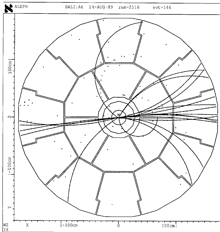
Рис. 4.60: r\phi проекция электрон-позитронной аннигиляции во времяпроекционной камере детектора ALEPH [270,271].
