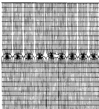
Рис. 4.26: Силовые линии поля и эквипотенциали в многопроволочной пропорциональной камере. Четко просматривается влияние незначительного сдвига одной из анодных проволочек на качество поля [51,182].
