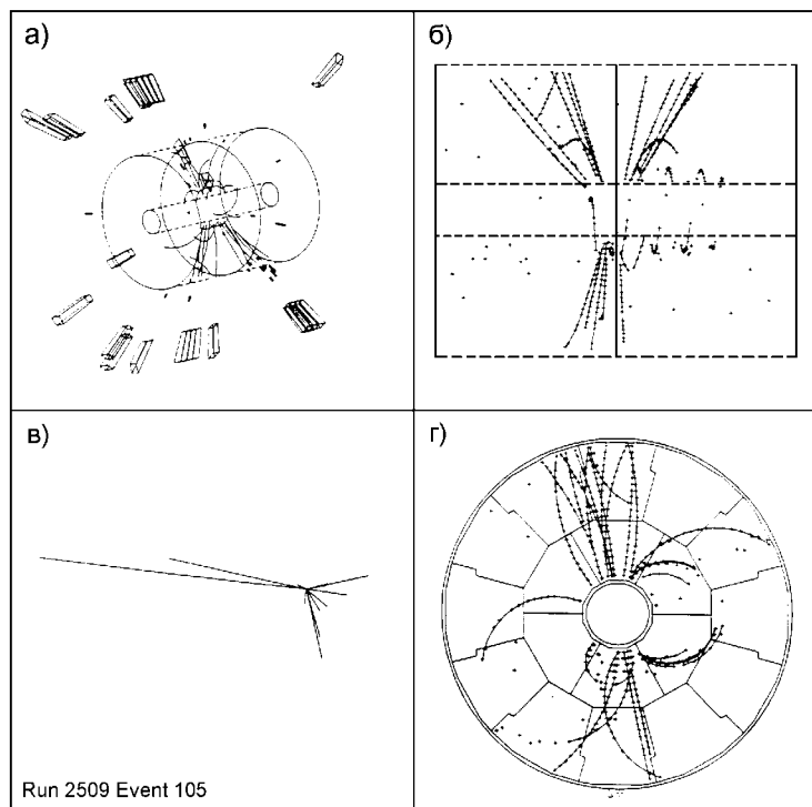
Рис. 11.22: Реконструкция адронного распада Z^0 в детекторе ALEPH: а) трехмерный вид с треками в ВПК и энергосделением в калориметрах; б) rz -проекция в ВПК; в) импульсная диаграмма. Длина линий пропорциональна импульсу частиц; д) r\varphi -проекция в ВПК [270].
