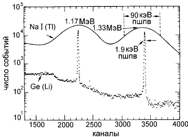
Рис. 7.1: Сравнение измерений спектра фотонов от источника ^{60}\text{Co} , полученных с помощью \text{NaI}(\text{Tl}) -сцинтиллятора и \text{Ge}(\text{Li}) -твердотельного детектора [479].
