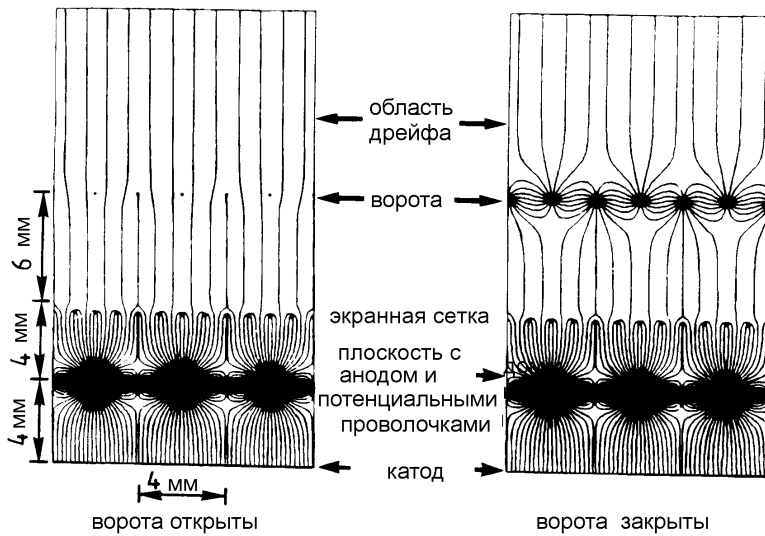
Рис. 4.59: Принцип работы «ворот» времяпроекционной камеры детектора ALEPH [270].
