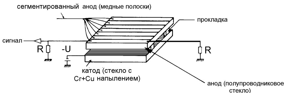
Рис. 5.21: Принцип работы плоской искровой камеры [1,425]. Во многих случаях катод покрыт либо полупроводящим материалом, либо веществом с высоким удельным объемным сопротивлением.
