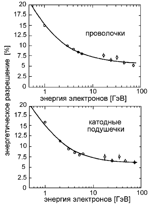
Рис. 7.29: Разрешение по энергии для электронов в медном калориметре на стримерных трубках [522].
