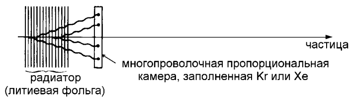
Рис. 6.22: Принцип работы детектора переходного излучения.
