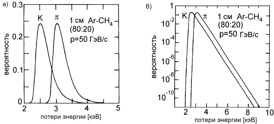
Рис. 6.31: Потери энергии пионов и каонов с импульсом 50 ГэВ/с в аргон-метановом слое толщиной 1 см в а) линейном и б) полулוגарифмическом масштабах.
