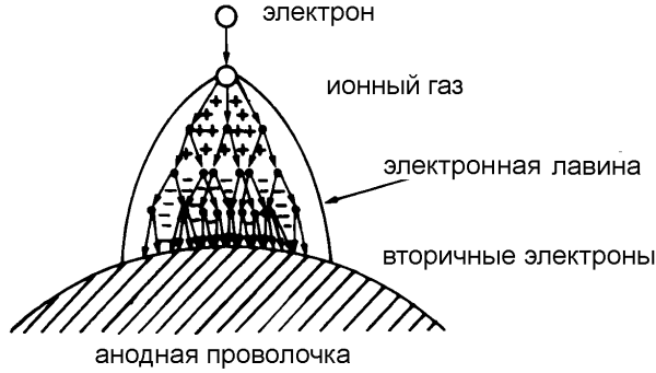
Рис. 4.9: Схема образования лавины на анодной проволочке в пропорциональном счетчике. Каплеобразная лавина образуется за счет боковой диффузии.
