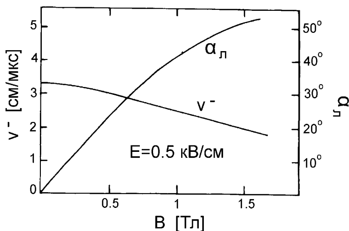
Рис. 1.21: Зависимость скорости дрейфа электрона v^- и угла Лоренца \alpha_L от магнитного поля при низкой напряженности электрического поля (0.5 кВ/см) в газовой смеси аргона (67%), изобутана (30%) и метилала (2.5%) [51,95].
