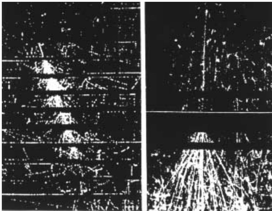
Рис. 4.70: Два электромагнитных каскада, инициированных мюонами космических лучей в многопластинчатой камере Вильсона [312,313].
