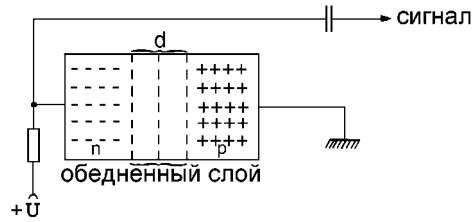
Рис. 7.3: Принцип действия (p-n) -полупроводникового счетчика (показаны лишь свободные носители заряда).
