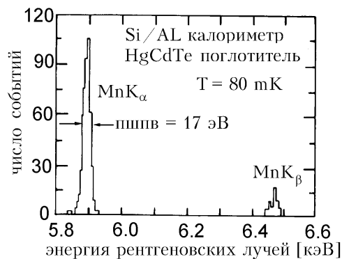
Рис. 7.14: Амплитудное распределение рентгеновских лучей с энергией 5.9 кэВ и 6.47 кэВ от K_{\alpha} - и K_{\beta} -линий (марганец) в болометре, состоящем из HgCdTe-поглотителя и Si/Al-калориметра. K_{\alpha} -линия соответствует переходу с L- на K-оболочку, K_{\beta} -линия — переходу с M- на K-оболочку [493].
