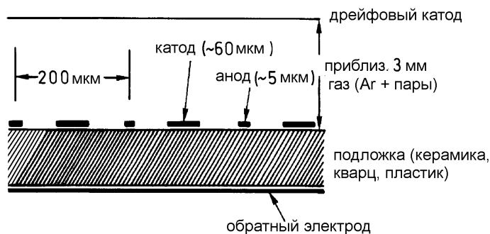
Рис. 4.30: Схематическая конструкция микрополоскового газового детектора.
