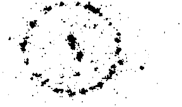
Рис. 6.19: Черенковское кольцо, образованное электроном с энергией 5 ГэВ [457].
