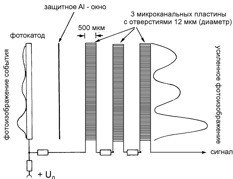
Рис. 5.7: Принцип работы фотоумножителя с трехступенчатой канальной пластиной.
