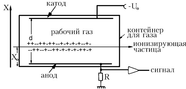
Рис. 4.1: Принцип работы плоской ионизационной камеры.
