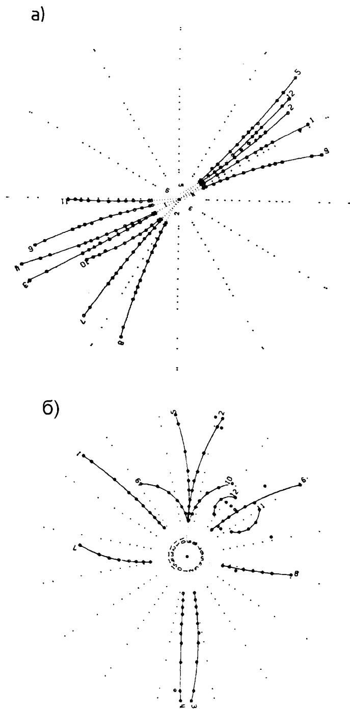
Рис. 4.47: Многотрековые события электрон-позитронного взаимодействия, измеренные в центральном детекторе PLUTO.
