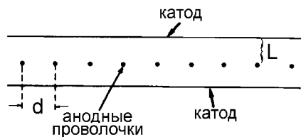
Рис. 4.24: Схематическое изображение конструкции многопроволочной пропорциональной камеры.
