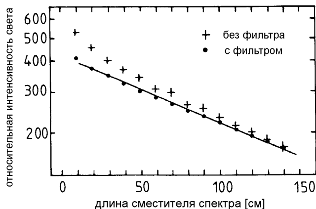
Рис. 5.12: Поглощение света в сместителе спектра (BBQ; стержень толщиной 3 мм) [402].
