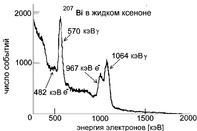
Рис. 7.12: Энергетический спектр конверсионных электронов и \gamma -лучей от изотопа ^{207}\text{Bi} в жидкоксероносовой камере [421].
