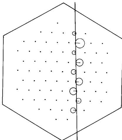
Рис. 4.51: Пример пролета одной частицы через многопроволочный дрейфовый модуль. Кружками обозначены измеренные времена дрейфа для сработавших проволочек. Трек частицы представляет собой общую касательную ко всем дрейфовым кружкам [259].
