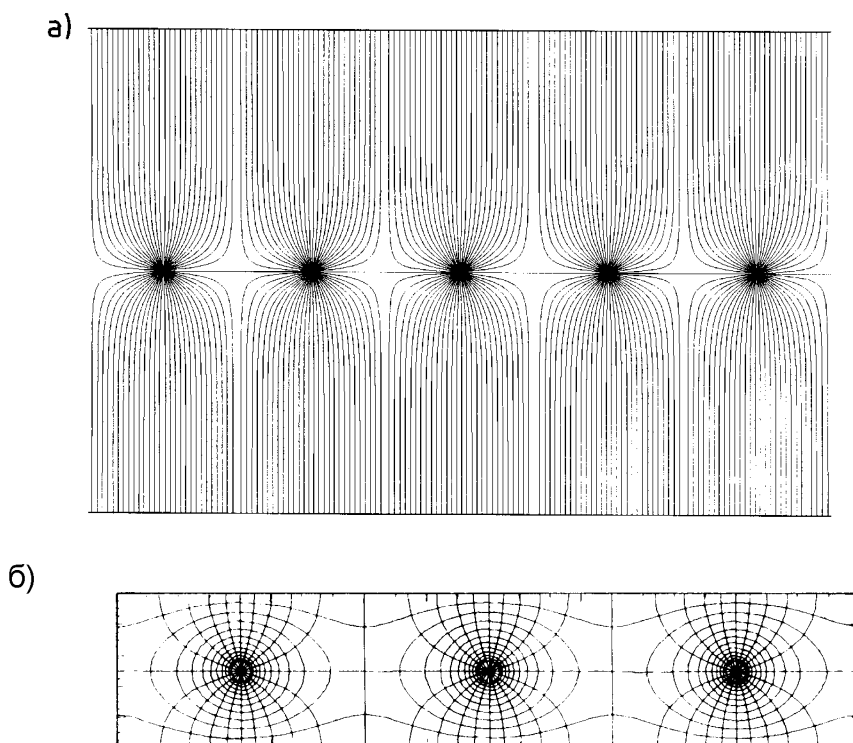
Рис. 4.25: Силовые линии поля в пропорциональной камере с а) пятью [184] и б) тремя проволочками (показаны также эквипотенциалы [183]).
