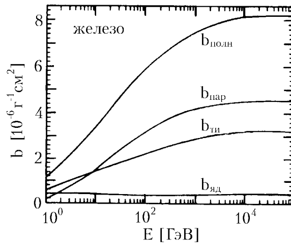
Рис. 1.5: Зависимость параметра b от энергии для мюонов в железе. Приведены частичные потери энергии на прямое рождение электрон-позитронных пар, ( b_{\text{пар}} ), тормозное излучение ( b_{\text{ги}} ) и фотоядерные взаимодействия ( b_{\text{яд}} ), а также их сумма ( b_{\text{полн}} ) [59].
