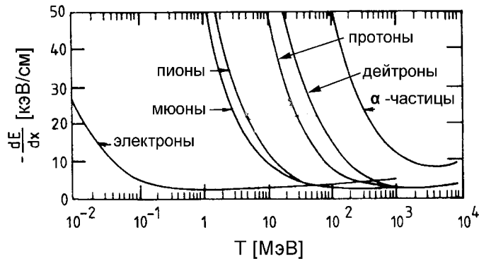
Рис. 1.2: Энергетические потери для различных частиц в воздухе [37].
