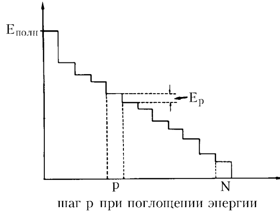
Рис. 1.4: Потери энергии за N дискретных шагов с передачей энергии E_p на p -ом шаге [54].
