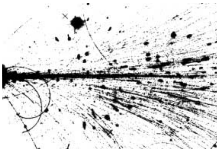
Рис. 4.74: Фотография взаимодействия тяжелых ионов ^{32}\text{S} с неподвижной золотой мишенью при энергии пучка 6400 ГэВ [319,321].
