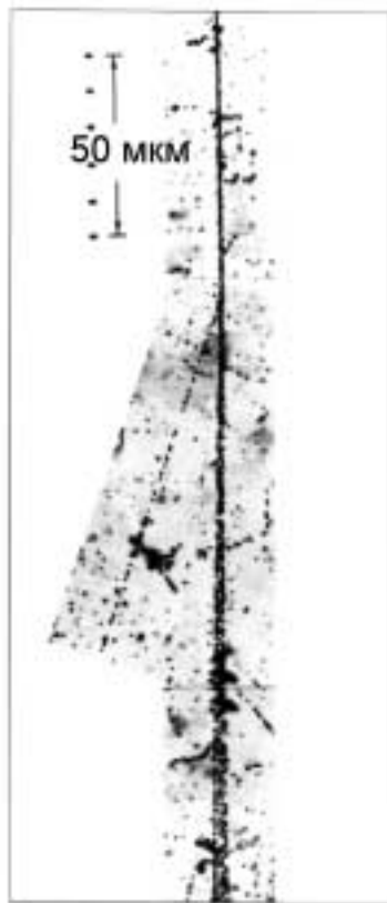
Рис. 4.93: Космическое ядро углерода сталкивается с протоном в ядерной эмульсии. Ядро углерода распадается на три \alpha -частицы. Протон отдачи рассеивается влево ([351], приведено в [301]).
