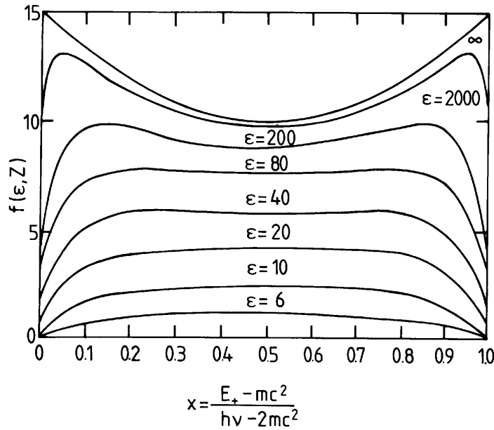
Рис. 1.13: Форма функции распределения энергии f(\epsilon, Z, x) с параметром \epsilon = E_{\text{пар}}/m_e c^2 . Полное сечение рождения пар дается площадью под соответствующей кривой в единицах Z(Z+1) \propto r_e^2 [37,71,72].
