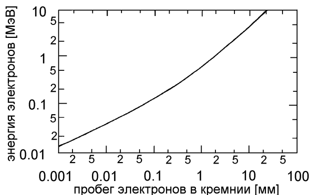
Рис. 7.7: Соотношение энергия-пробег для электронов в кремнии [487].
