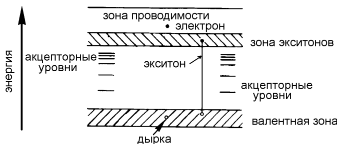
Рис. 5.9: Энергетические зоны в кристаллах.
