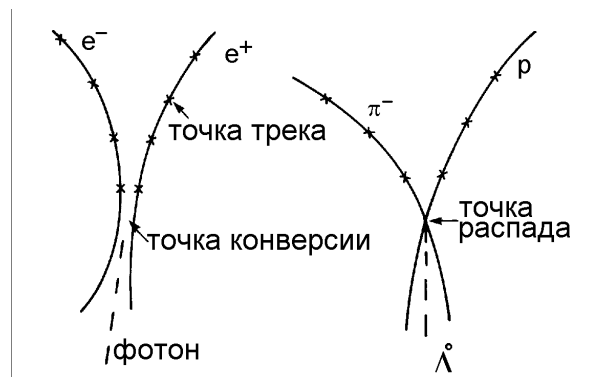
Рис. 10.4: Картина конверсии фотона и \Lambda^0 -распад.
