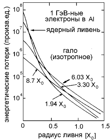
Рис. 7.22: Поперечные ширины электромагнитных ливней как функция их глубины [505,508,514].
