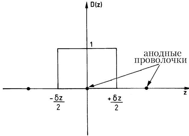
Рис. 2.1: Схема определения дисперсии прямоугольного распределения.
