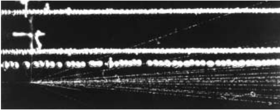
Рис. 4.68: «Старые» и «новые» треки в пузырьковой камере с высоким разрешением [305].
