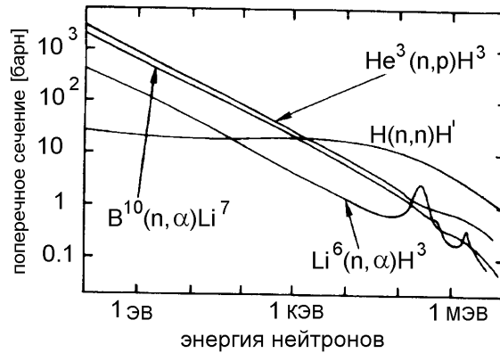
Рис. 6.1: Зависимость сечения реакций, индуцированных нейтронами, от их энергии (1 барн = 10^{-24} \text{ см}^2 ) [442].
