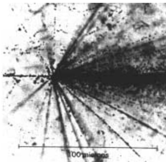
Рис. 4.91: Взаимодействие иона серы с энергией 6.4 ТэВ с ядром в фотографической эмульсии [354].
