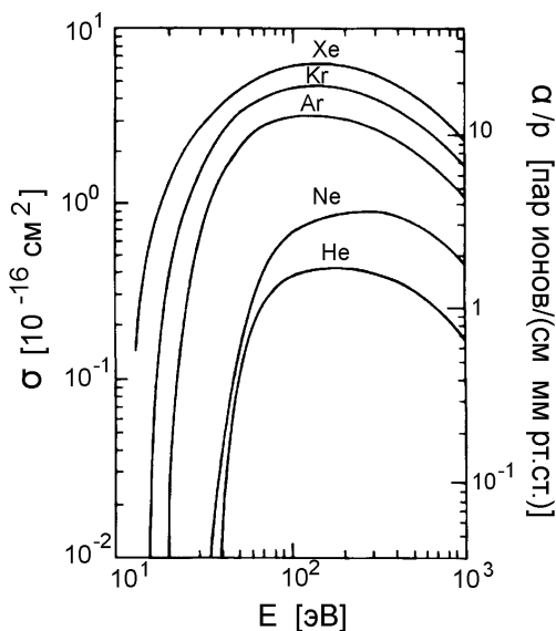
Рис. 4.5: Энергетическая зависимость фотоионизации и ее сечения за счет столкновений [104,139,140].
