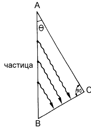
Рис. 6.8: Простое геометрическое определение черенковского угла.
