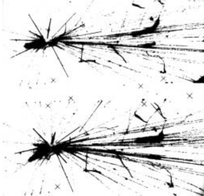
Рис. 4.75: Стереорафическое изображение протон-антипротонного взаимодействия с энергией в системе центра масс 900 ГэВ (UA5-эксперимент) [320,322].
