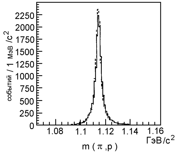
Рис. 10.6: Инвариантная масса m(p, \pi^-) для отбора \Lambda^0 -кандидатов после кинематической реконструкции. Сплошная линия показывает распределение экспериментальных данных, пунктирная — монте-карловское моделирование.
