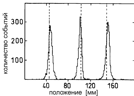
Рис. 4.20: Распределения скоростей счета 5.9 кэВ-ных фотонов, влетающих в разных местах вдоль анодной проволоки в стримерной трубке [165].
