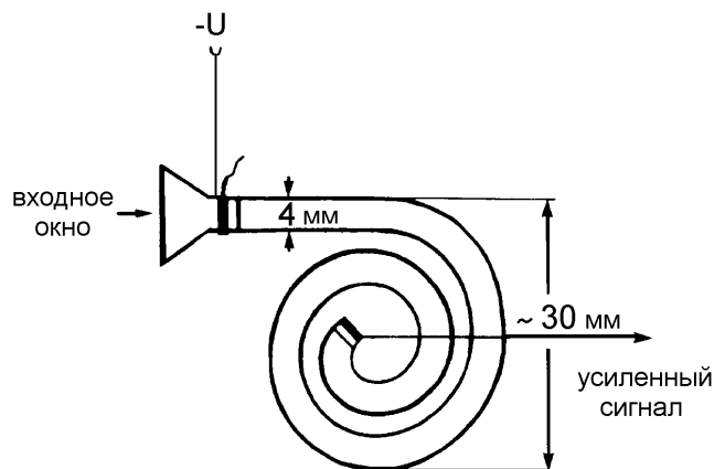
Рис. 5.8: Одиночный канальный электронный умножитель [379].
