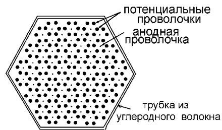
Рис. 4.49: Схематическое изображение многопроволочного дрейфового модуля. В этой гексагональной структуре каждая анодная проволочка окружена шестью потенциальными. В одном контейнере диаметром 30 мм, изготовленном из материала на основе углеродистого волокна, размещено семьдесят дрейфовых ячеек [259].
