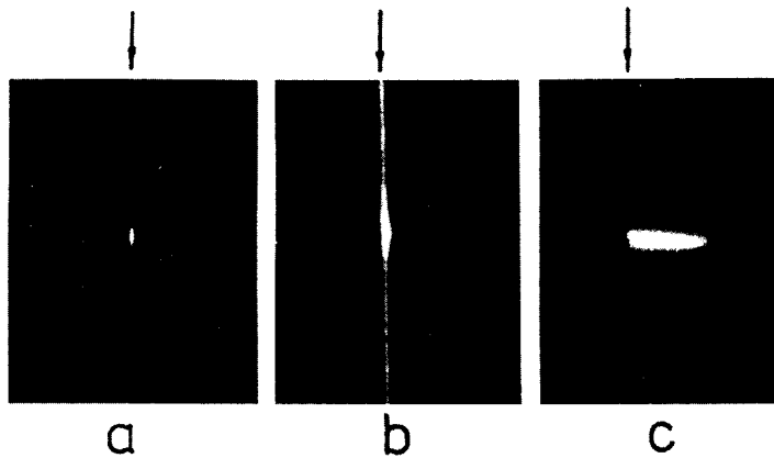
Рис. 4.17: Газовые разряды в (а) пропорциональном счетчике, (б) счетчике Гейгера и (в) самогасящейся стримерной трубке; стрелками указано положение анодной проволоочки [166].
