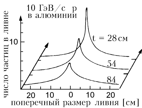
Рис. 7.40: Поперечный профиль ливня от протонов с импульсом 10 ГэВ/с в алюминии [559].
