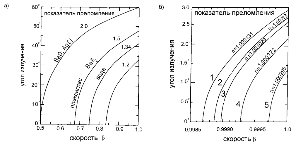
Рис. 6.9: Зависимость черенковского угла от скорости частицы в а) различных материалах и б) газах при различных показателях преломления [71]: 1 — изобутан, 2 — фреон (газообразный при 26°С и 760 мм рт. ст.), 3 — пропан, 4 — этан, 5 — воздух.
